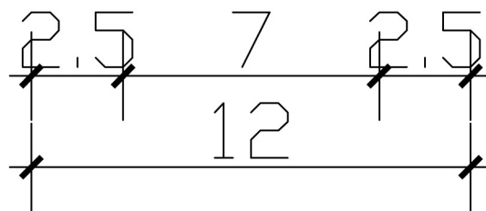
C-C 道路横断面
