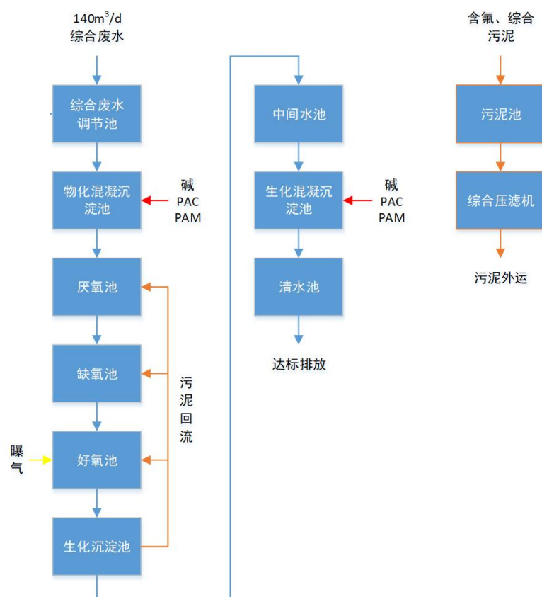
图4-1 生产废水处理工艺流程图
