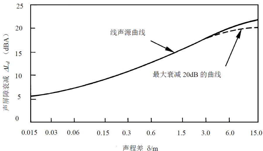
图 6-2 无限长声屏障衰减量与声程差关系图
