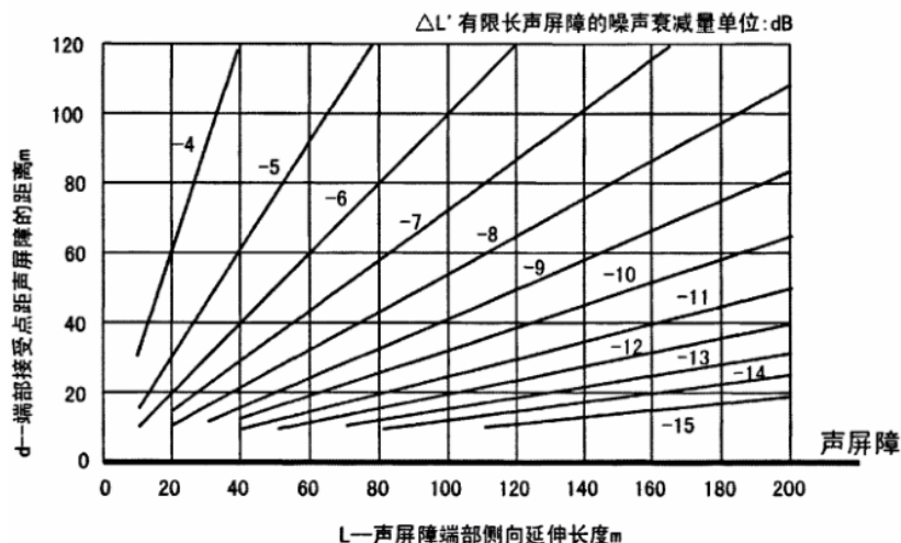
图 6-6 声屏障侧向延伸长度与噪声衰减量关系图
