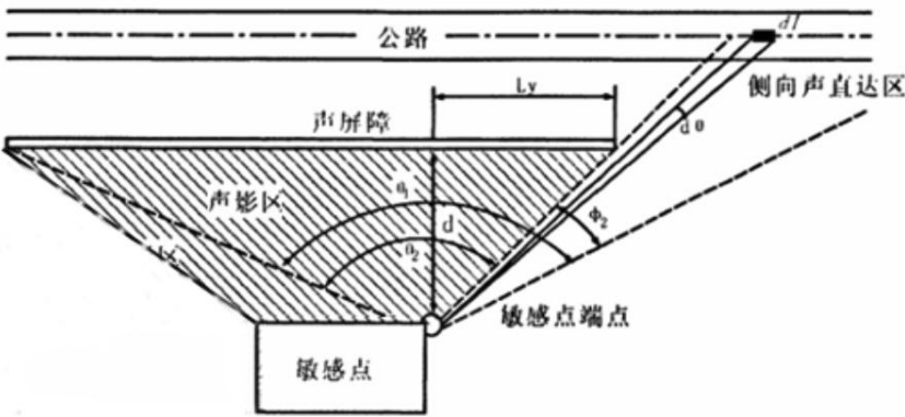
图 6-5 声屏障侧向延伸长度 L_y 平面图
