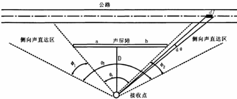
图 6-4 有限声屏障噪声衰减量计算示意图
