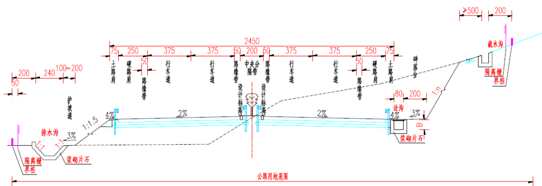
图2-1 现状标准横断面
