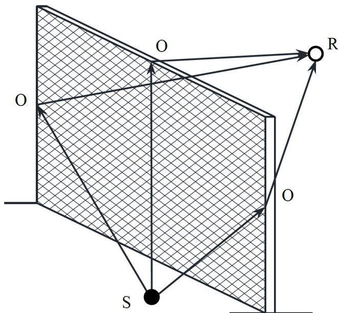
图 5-4 有限长声屏障传播路径
