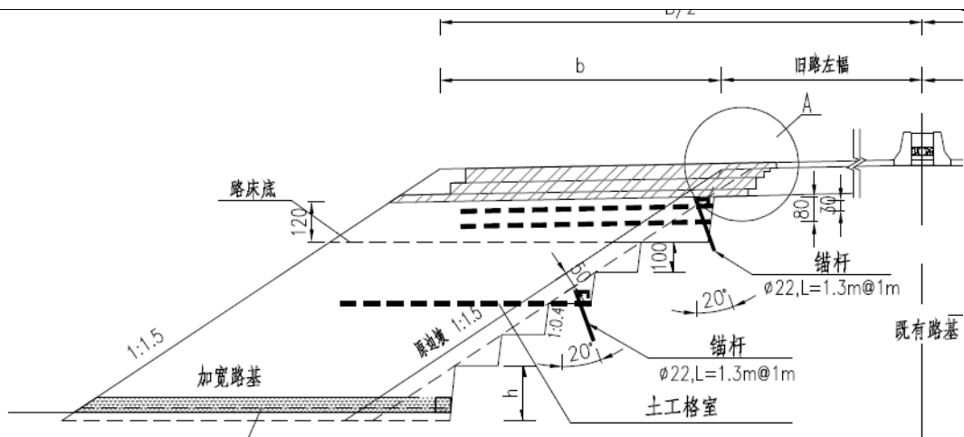
图 2-3 非软基路段路基拼接示意图
