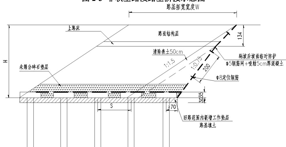
图 2-4 软基路段路基拼接示意图
