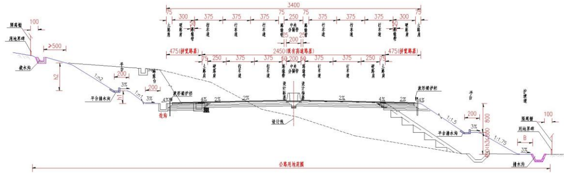
图 2-2 扩建后路基标准断面图（24.5m 扩建为路基宽度 34m）
