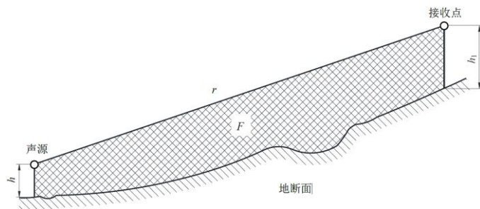
图 5-2 估计平均高度 h_m 的方法图
