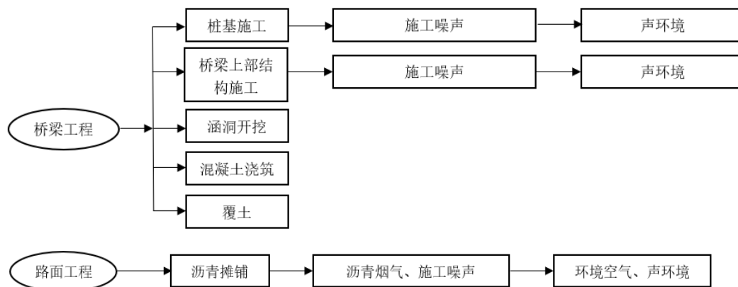
图 2-8 施工期公路施工工艺及排污点位示意图
