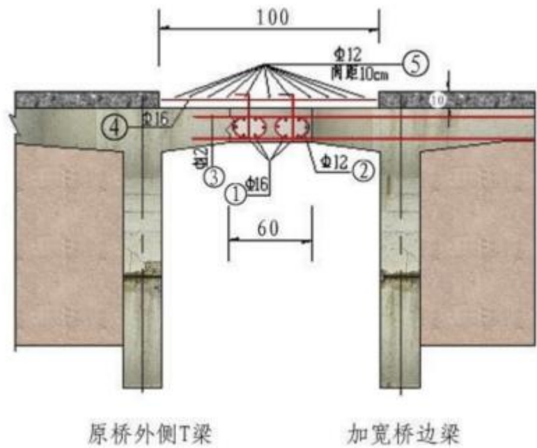
图 2-7 T 梁拼接推荐方案
