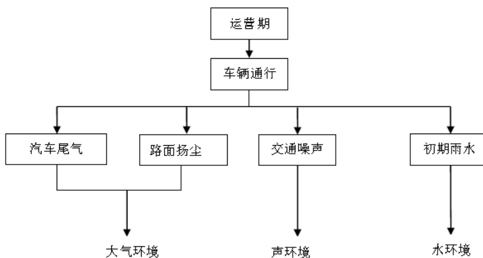
图 2-9 运营期公路工程排污点位示意图
