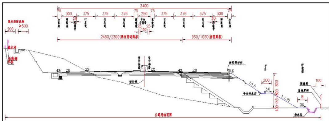
图2-2 整体式六车道34m标准横断面形式
