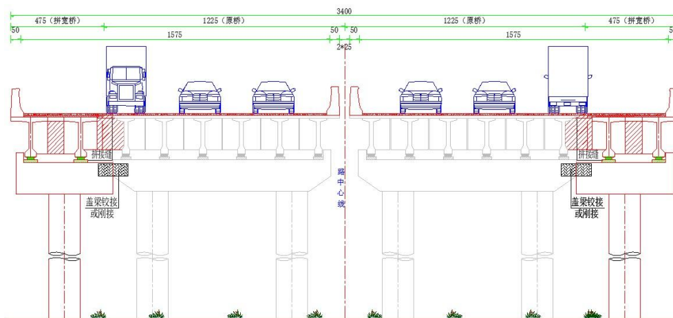
图 2-6 两侧拼宽扩建标准横断面
