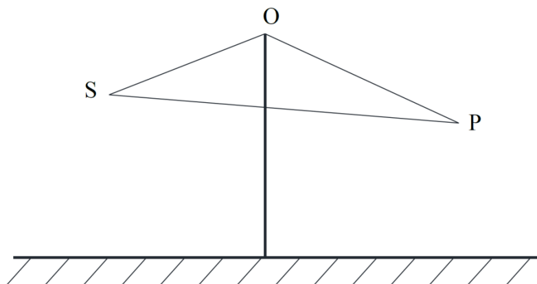
图 5-3 无限长声屏障示意图
